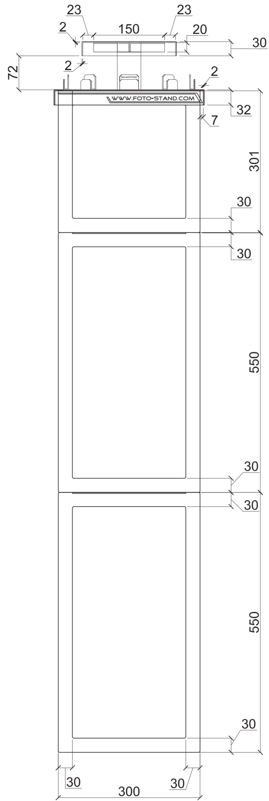
2 ELEWACJA KONSTRUKCJA 1 Scale: 1:5
