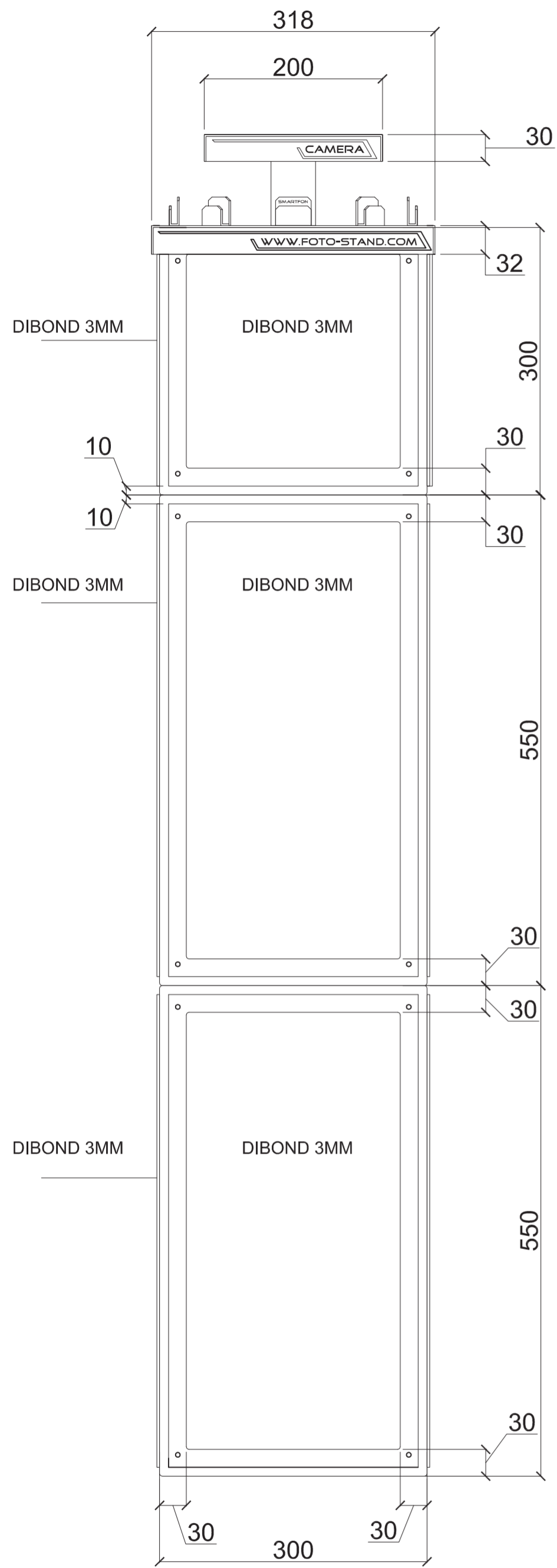
1 ELEWACJA 1 Scale: 1:5
